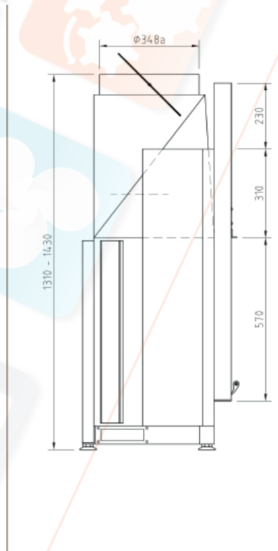
Боковое изображение М 1:20
